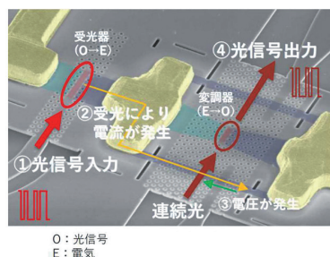
【光トランジスタの概要図】
